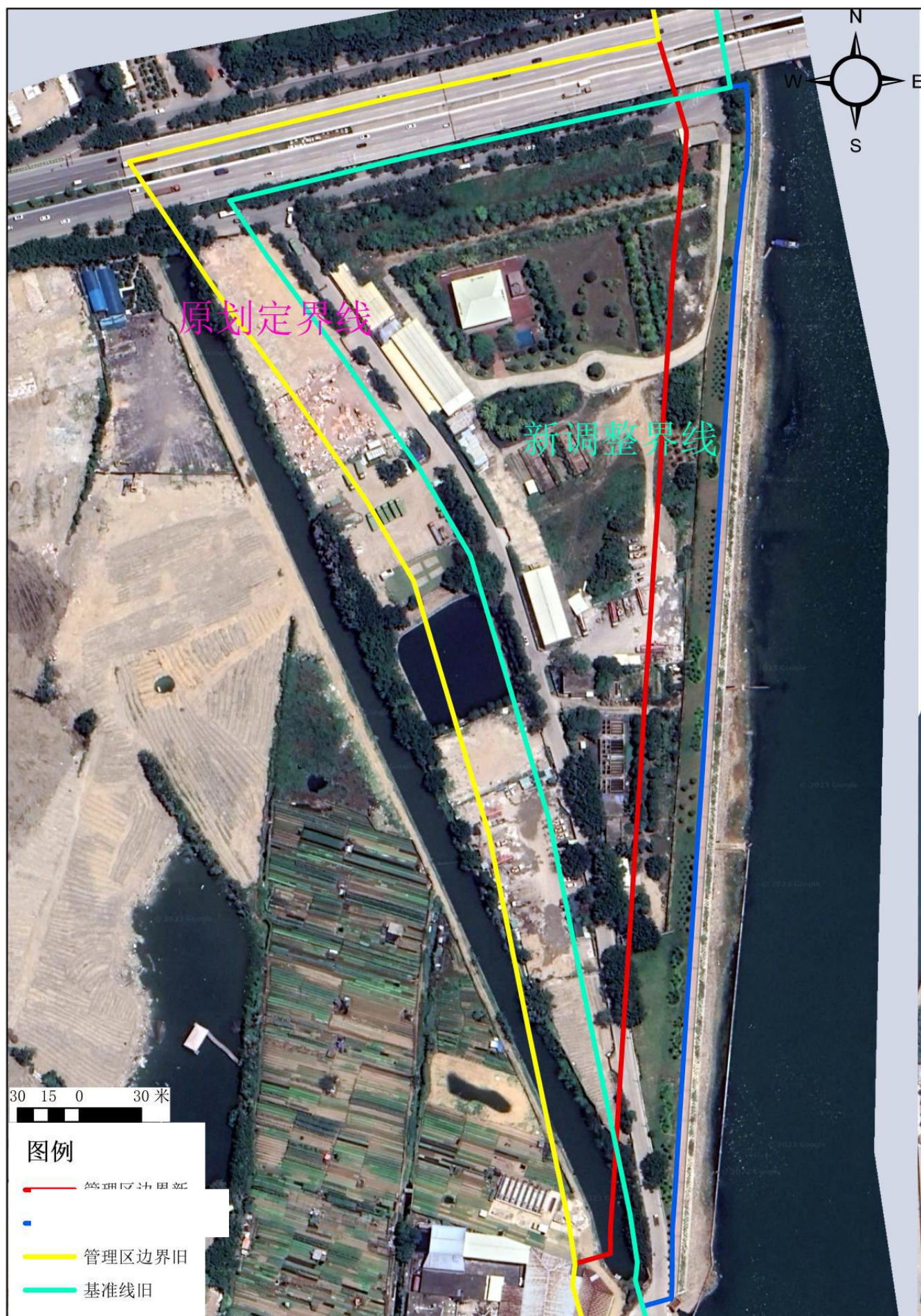
龙湖区新津河右岸东坝仔堤段河道管理范围划定调整前后对比图
