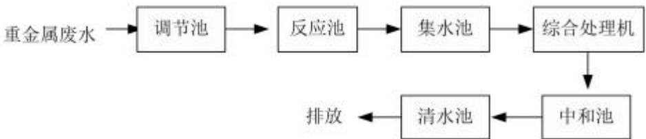
图 3.3-1 超声生产废水预处理工艺流程图
